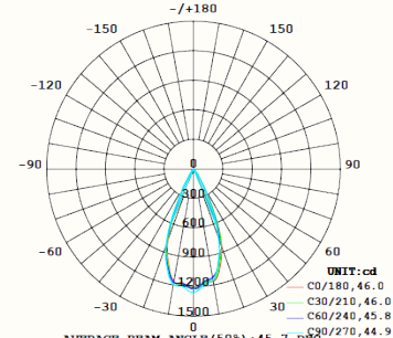
50° Linse 38906
