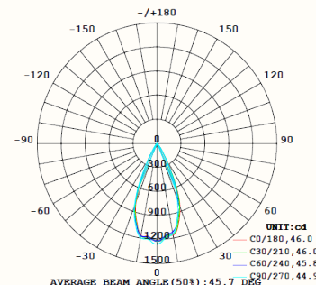
50° Linse 38906
