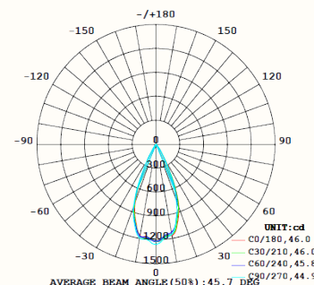
50° Linse 38906
