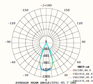
50° Linse 38906
